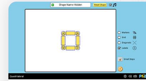
Quadrilateral
